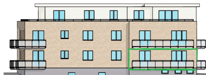
SÜDANSICHT
